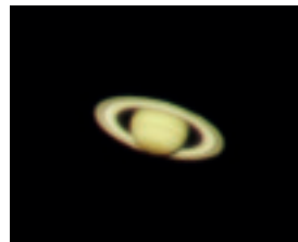
Planeten Saturnus, fotograferad från Åkesta
