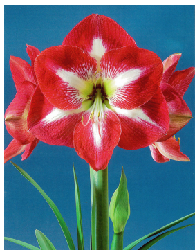
Monte Carlo
